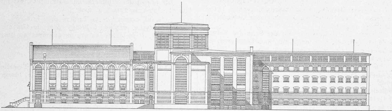
SEITENSICHT
