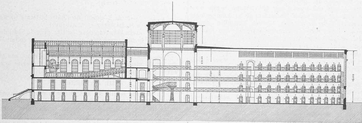
SCHNITT A-B
