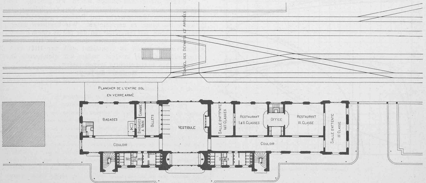
Plan du rez-de-chaussée. Echelle: 1 cm = 6 m.
