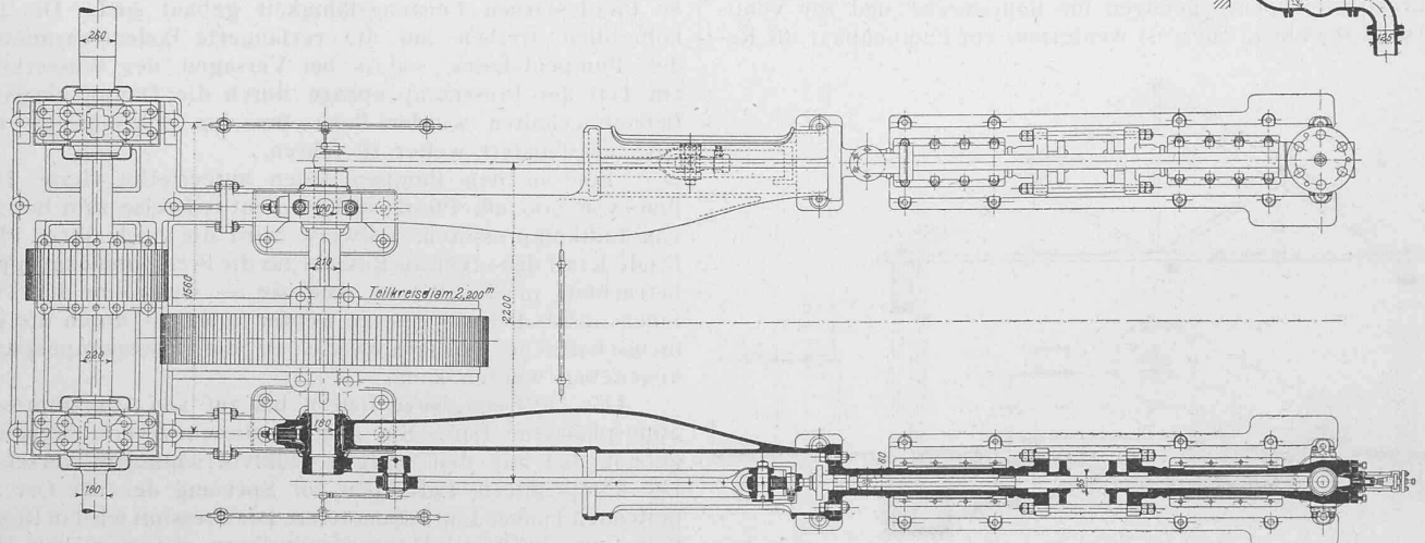
Abb. 64. Hochdruckpumpenpaar (grösseres Modell) mit Vorgelege. — Masstab 1 : 50.
