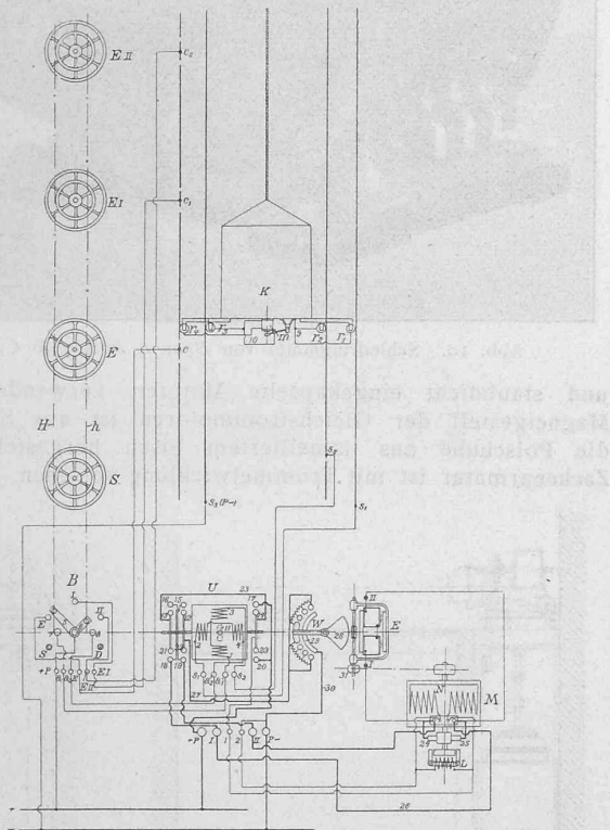
Abb. 7. Schema der selbsttätigen Stockwerk-Einstellvorrichtung der Elektrizitäts-A.-G. Schuckert & Cie.
