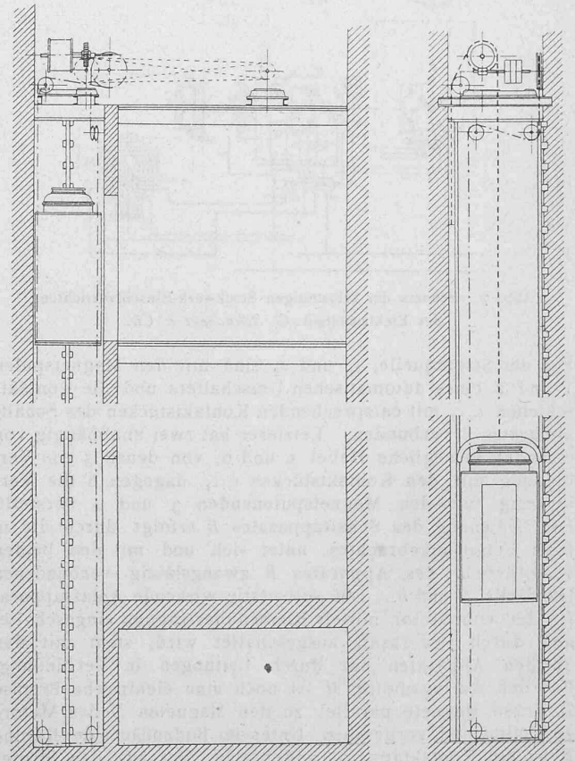
Abb. 11. Anordnung eines Personenaufzuges von Alfred Schindler in Luvern. — Aufrisse. Masstab 1:100.
