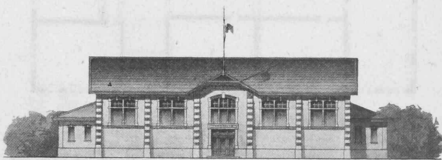
Turnhalle, Fassade gegen den Turnplatz. Masstab 1:500.
