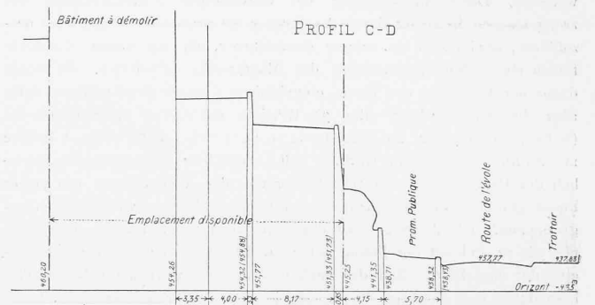
Querprofile. — Masstab 1 : 600.
