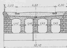
Querschnitte. — 1 : 300.
