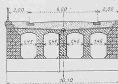
Querschnitte. — 1 : 300.
