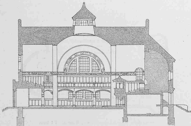
Längsschnitt. — Masstab 1 : 400.
