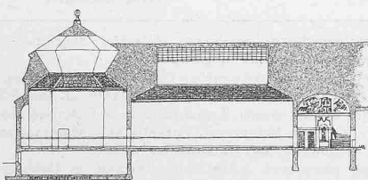
Schnitt I—II.
