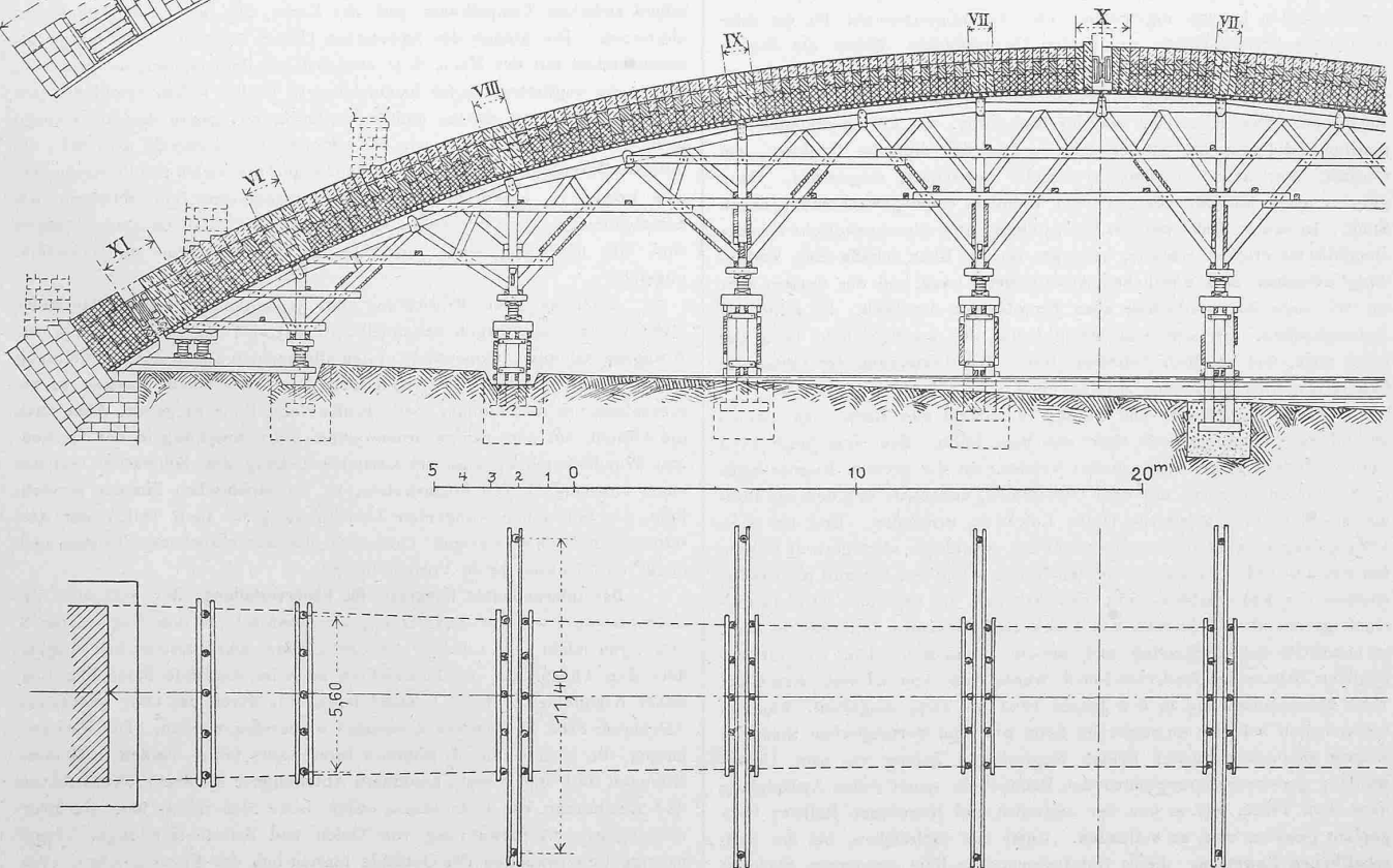
Abb. 3. Darstellung des Lehrgerüsts und der Ausführung des Gewölbemauerwerkes. — Längsschnitte und Grundriss. — Masstab 1 : 250.
