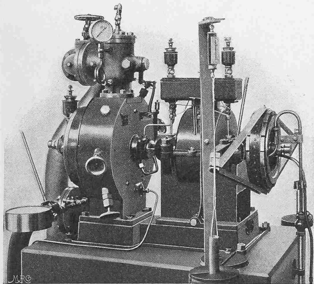
Abb. 17. 10 P. S.-de Laval-Dampfturbine.
