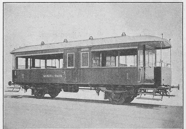
Abb. 6. Anhängewagen der Adhäsionsstrecke.
