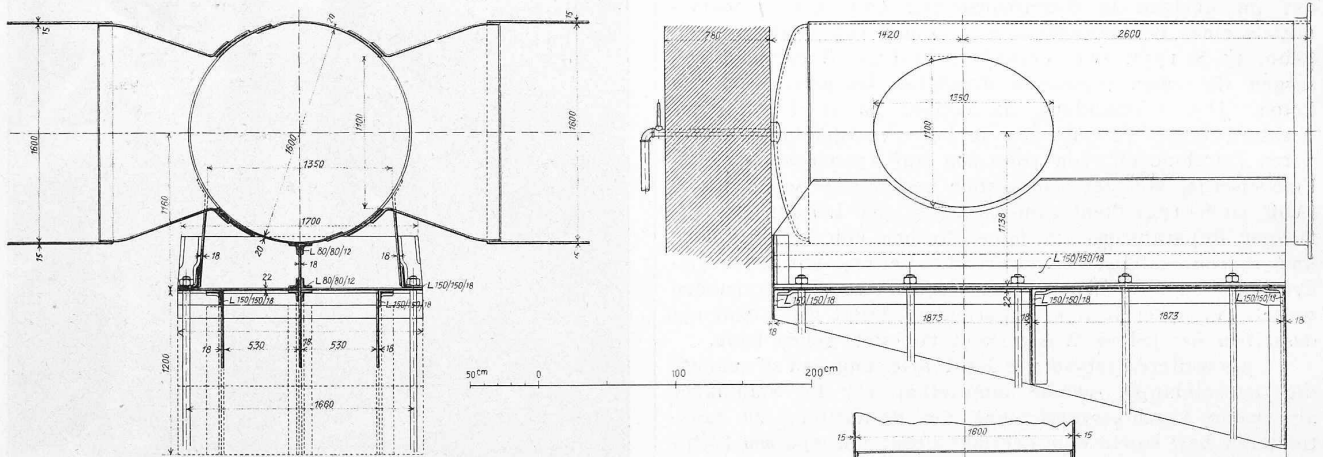
Abb. 31. Das T-Stück der Druckleitung beim Maschinenhaus. — 1:40.
