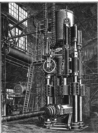
Dampfhdraulische Schmiedepresse. Stahlformguss bis zu 50 000 kg Stückgewicht.
