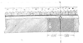
Querschnitt. — Masstab 1 : 250.
