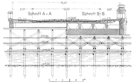
Querschnitt. — Masstab 1 : 250.
