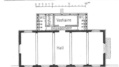
Ansicht und Grundriss der Turnhalle. — 1 : 600.
