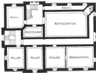
Kellergeschoss
