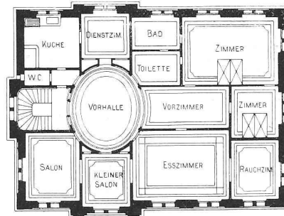
II. Obergeschoss
