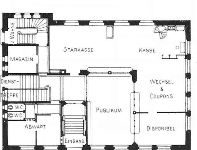
Erdgeschoss
