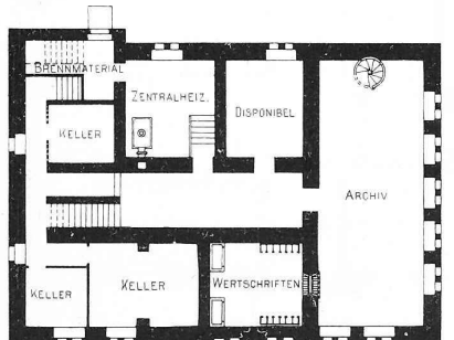
Kellergeschoss
