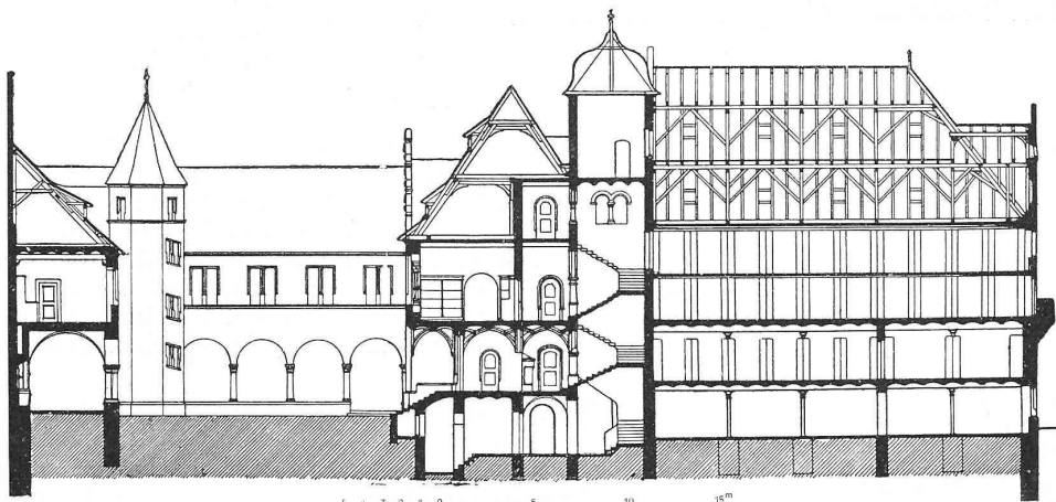
Abb. 42. Längsschnitt durch das Magazin- und das Verwaltungsgebäude des Staatsarchivs sowie durch den Hof an der Martinsgasse. — Masstab 1 : 400.
