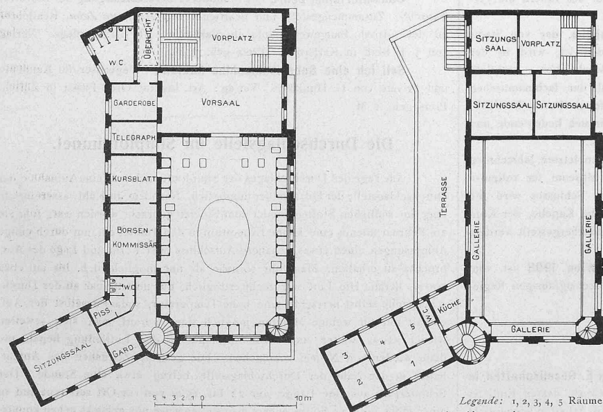
Grundrisse vom ersten und zweiten Obergeschoss. — Masstab 1:500.
