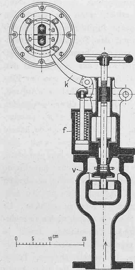
Abb. 6. Sicherheitsregulator mit Schnellschlussventil. Masstab 1 : 10.
