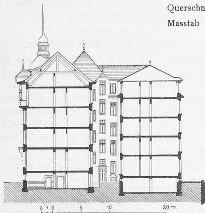
Querschnitt.
