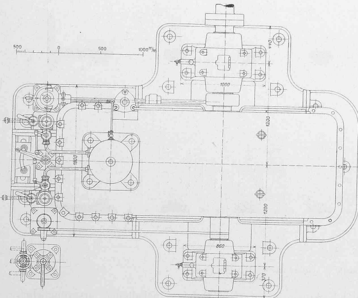
Abb. 45. Grundriss.
