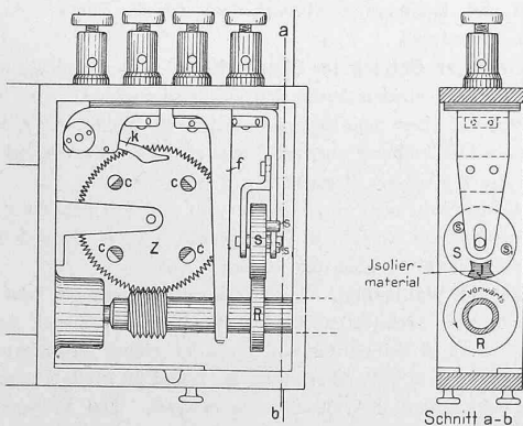
Abb. 8. Kontaktvorrichtung des Flügels Nr. 795. — Masstab 1 : 2. Legende: Z Zahnrad, c Kontaktstifte, f Zunge.
