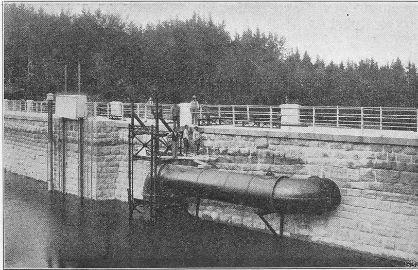
Abb. 3. Ansicht des Heberrohres an der Innenseite der Stauwand.
