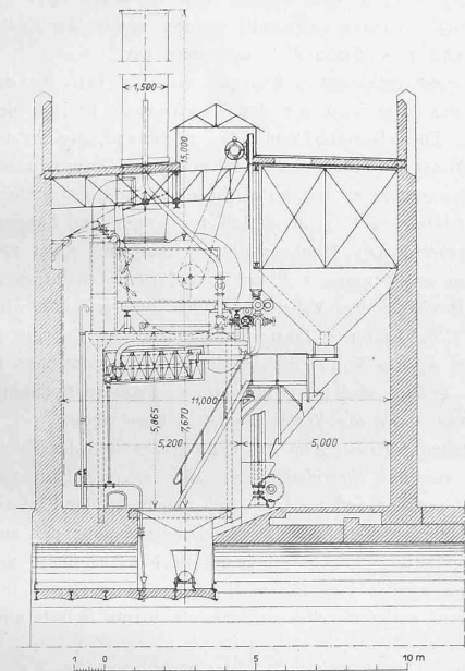
Abb. 47. Kesselhausquerschnitt. — 1 : 250.
