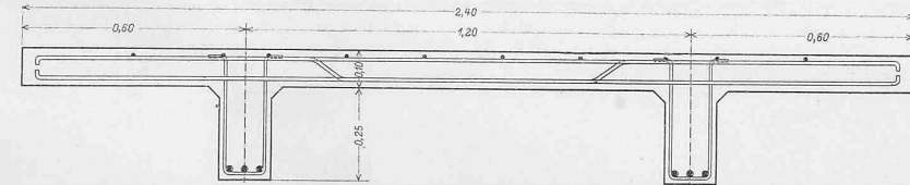
Abb. 13. Anordnung der Balkenpaare. — Masstab 1 : 20.
