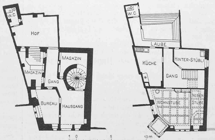
Abb. 3 u. 4. Grundrisse vom Hause «zur Stärke» in St. Gallen. — 1 : 300.
