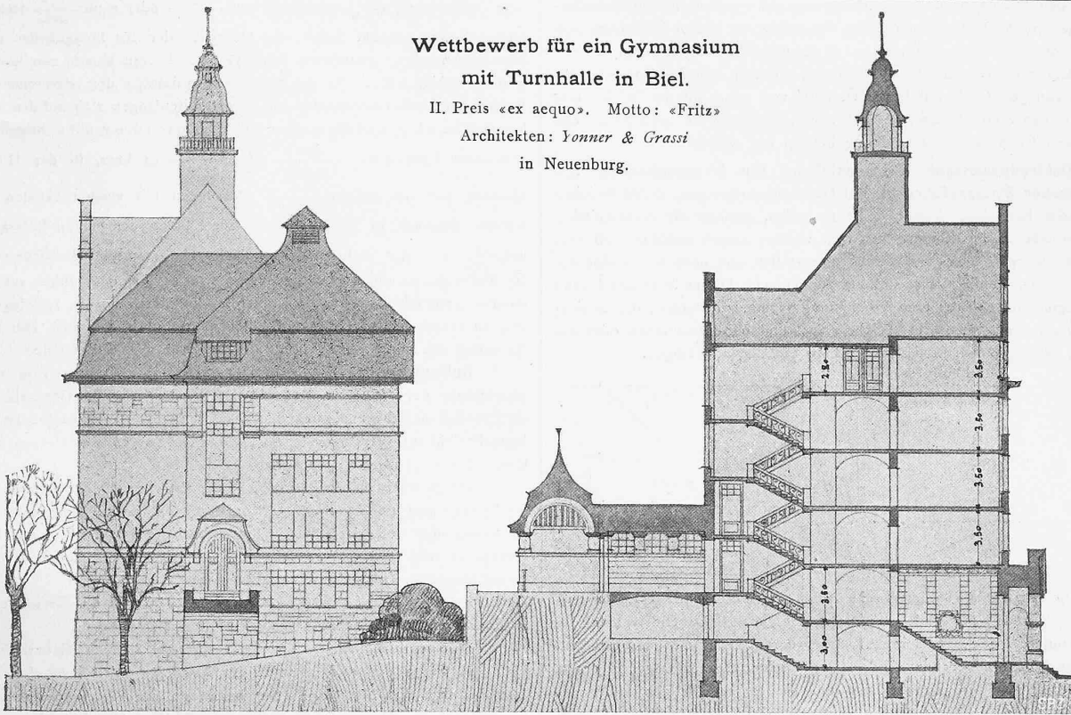
Seitenfassade und Querschnitt durch Haupteingang und Treppenhaus des Schulgebäudes. — Masstab 1 : 400.
