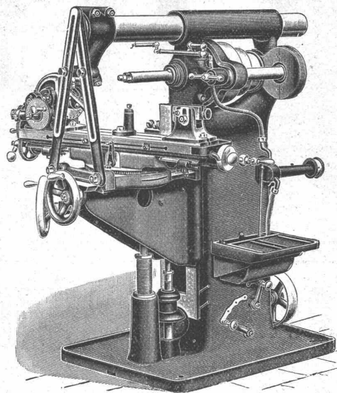
Universal-Fräsmaschine. No. 2.
