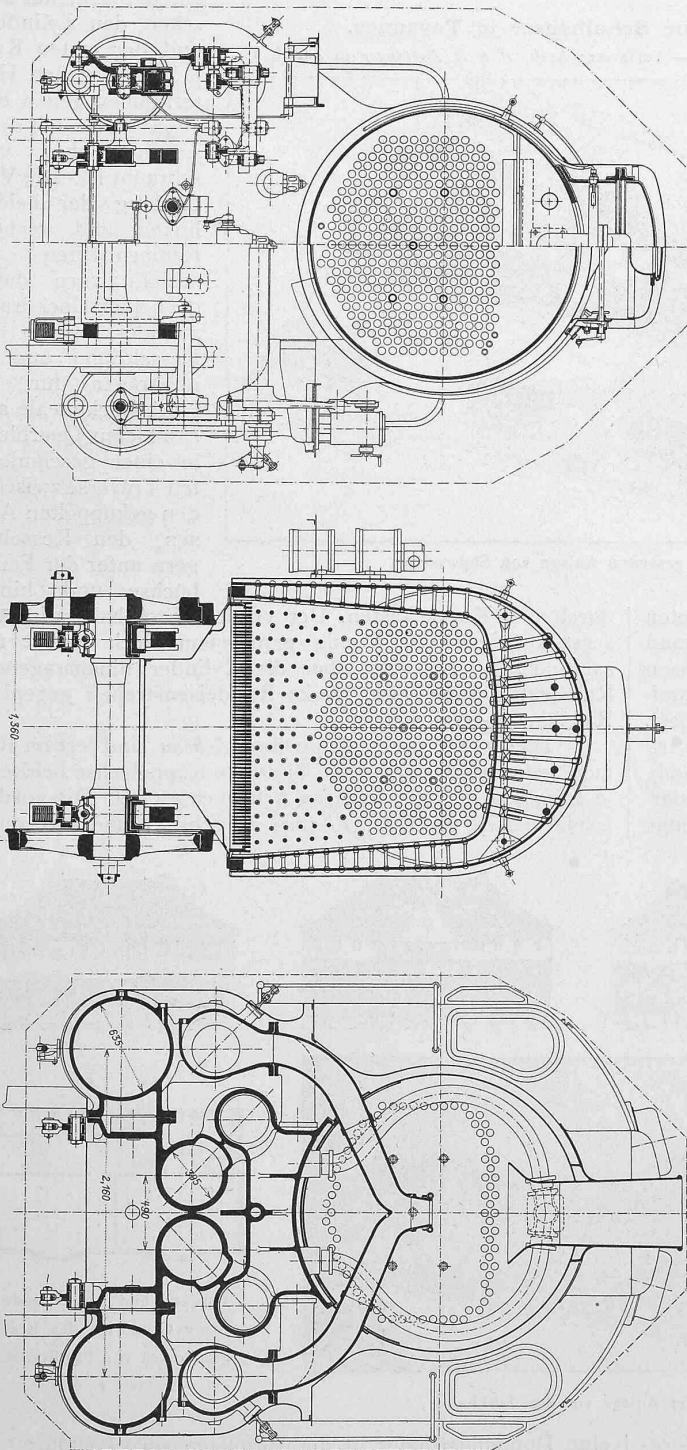
Abb. 4. Querschnitte der Lokomotive durch Kessel, Feuerbüchse und Zylinder. — Massstab 1 : 45.
