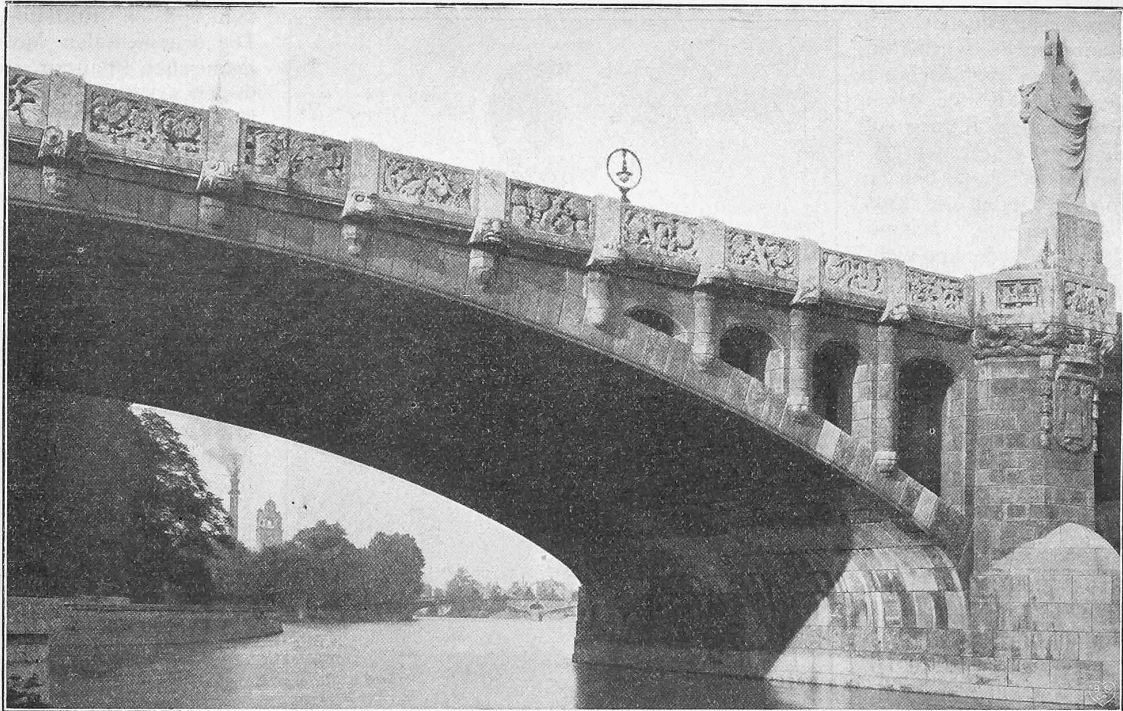
Abb. 2. Oestlicher Teil der Maximiliansbrücke in München. — Konstruktionsentwurf von Sager & Woerner .
