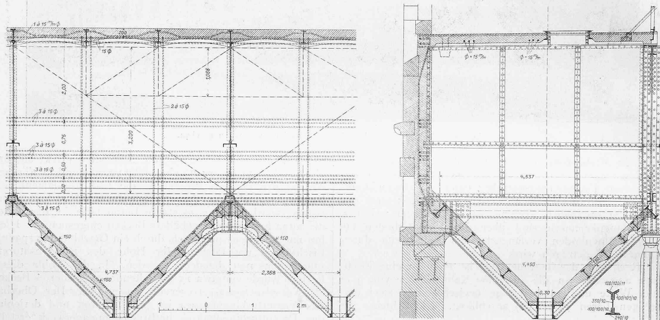
Abb. 21. Längenschnitt und Querschnitt eines Kohlenbunkers über dem Kesselhaus. — Masstab 1 : 75.
