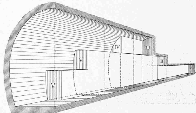
Abb. 3. Schematische Darstellung der Firstschlitzmethode.
