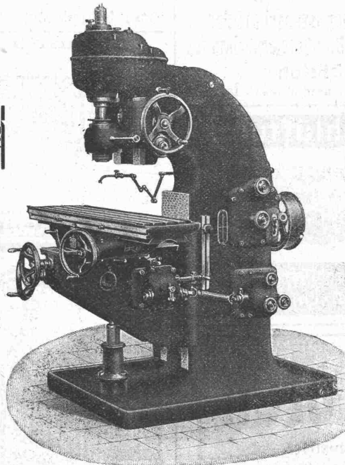
Vertikal-Fräsmaschine Nr. 3.
