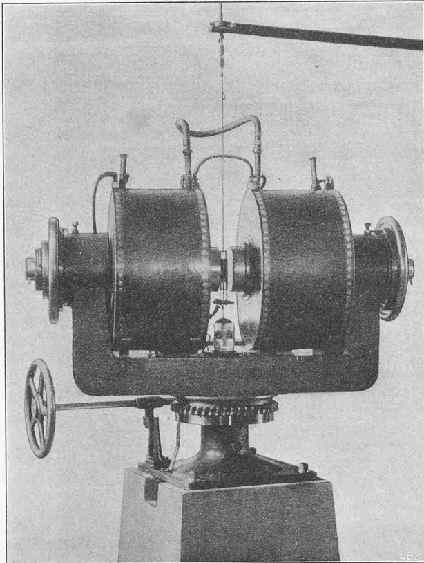
Abb. 3. «Elektromagnet Weiss» (grosses Modell) für 200 000 Ampèrewindungen im Physikal. Institut des eidg. Polytechnikums.
