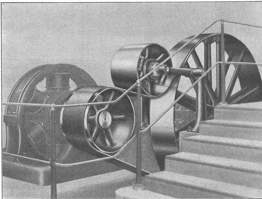
Spannrollentrieb mit Oelumlaufliefert für Generator-Antrieb 225 P. S. 500 mm breiter Doppelriemen.
