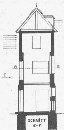
Geometrische Ansicht und Schnitte zu Projekt Nr. 7 für Typ D.
