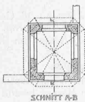
Geometrische Ansicht und Schnitte zu Projekt Nr. 7 für Typ D.
