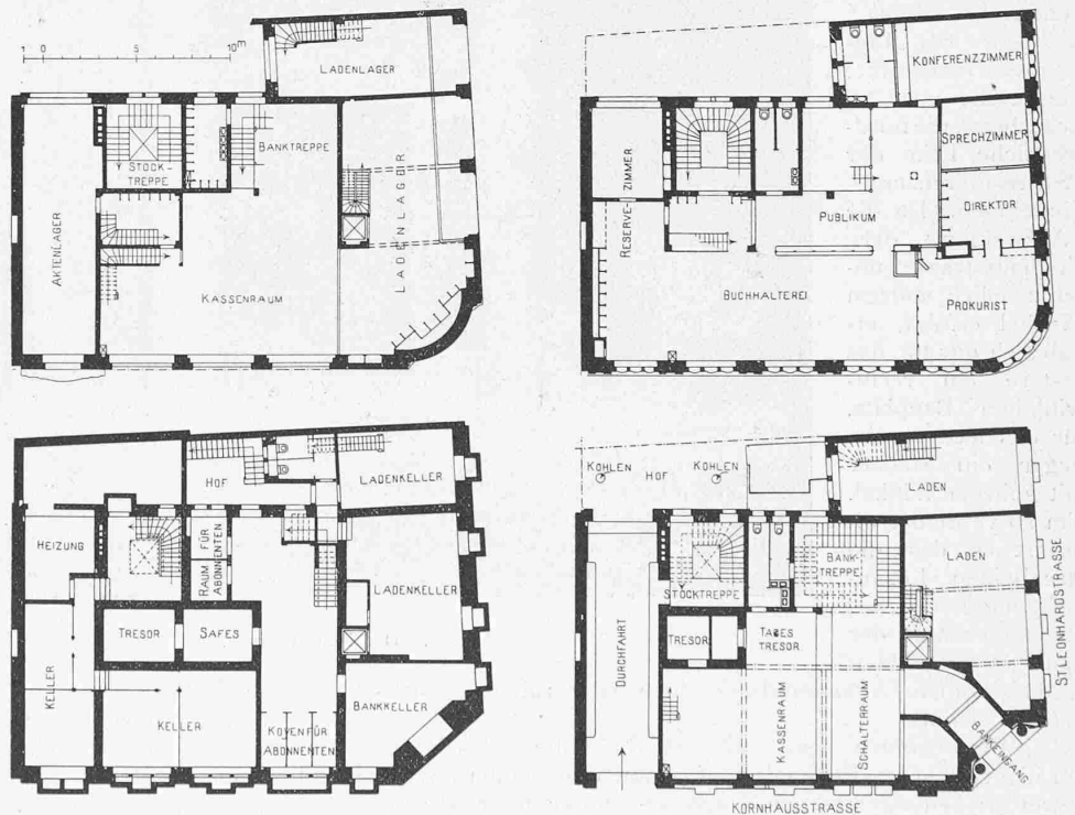
Abb. 1 bis 4. Grundrisse vom Untergeschoss, Erdgeschoss, Zwischengeschoss und I. Stock. Masstab 1 : 400.
