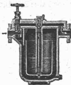
Dampfwasser-Ableiter.
