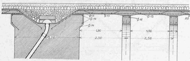
Längsschnitt g-g. — Masstab 1 : 100.
