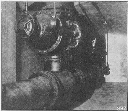
Abb. 26. Zweigleitung einer Maschinengruppe.
