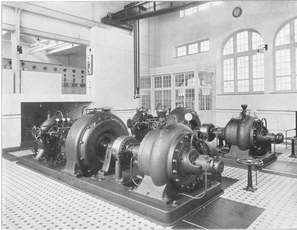
AKKUMULIERANLAGE DES ELEKTRIZITÄTSWERKES DER STADT SCHAFFHAUSEN MASCHINENSAAL
