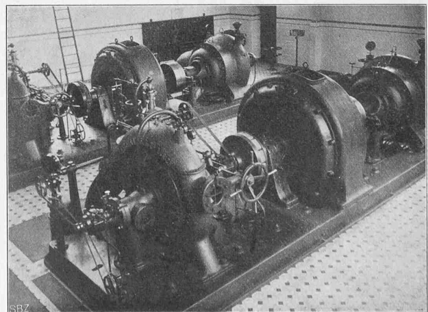
Abb. 25. Blick von der Schaltbühne auf die Maschinengruppen.
