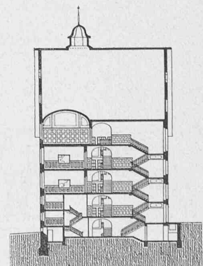
Schnitt. — Masstab 1:800.
