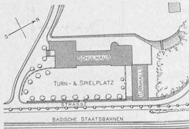
Lageplan. — Masstab 1 : 3000.
