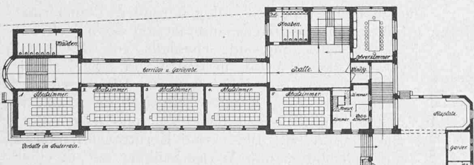
Hauptgeschoss, Untergeschoss u. Dachstock. — 1:800.
