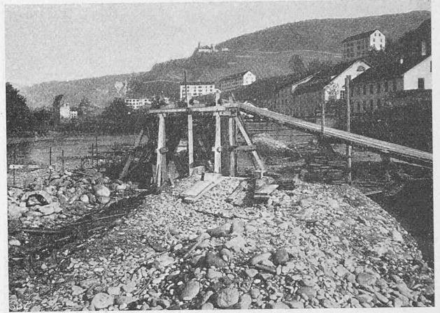
Abb. 22. Einschaltung eines 6 m-Eisenbeton-Senkkastens. (28. Oktober 1907.)
