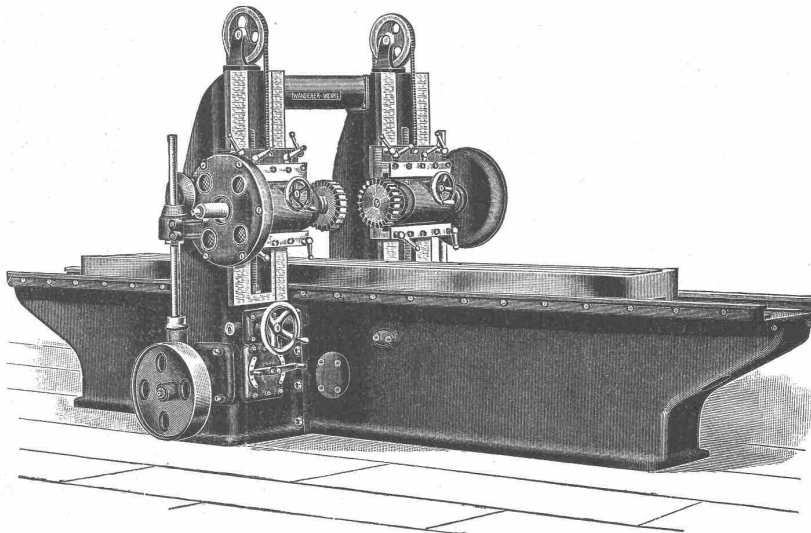
Doppel-Plan-Rapid-Fräsmaschine mit Einzelscheiben-Antrieb.
