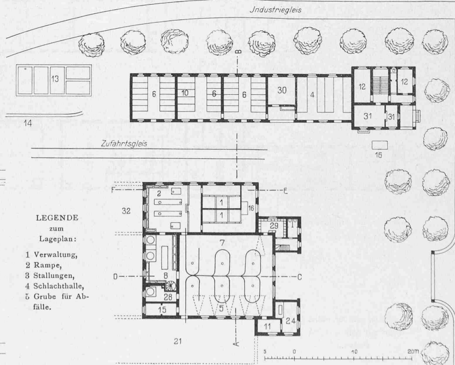
Grundriss und Schnitte. — Masstab 1:600,
