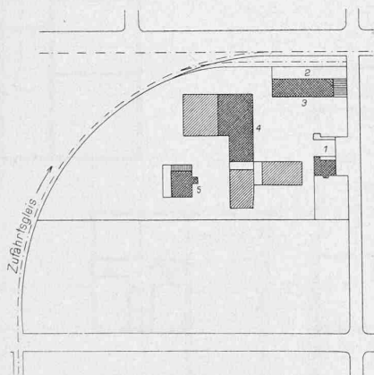
Lageplan. — Masstab 1:3000.
