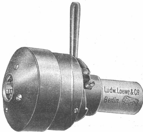
Gewindeschneidkopf R O S mit automatisch sich öffnenden Backen.
