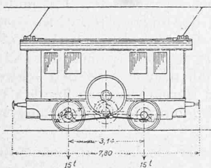
Abb. 1 und 2. Lokomotiven der Burgdorf-Thun-Bahn, gebaut 1899 und 1910, von Brown, Boveri &amp; Co., Baden. — Masstab aller Typenskizzen 1 : 200.
