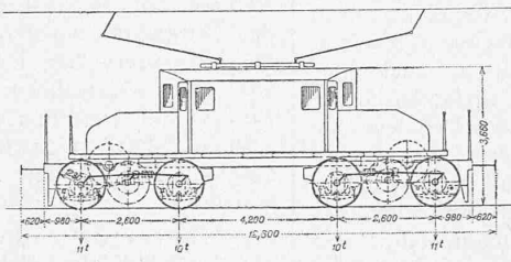
Abb. 1 und 2. Lokomotiven der Burgdorf-Thun-Bahn, gebaut 1899 und 1910, von Brown, Boveri &amp; Co., Baden. — Masstab aller Typenskizzen 1 : 200.
