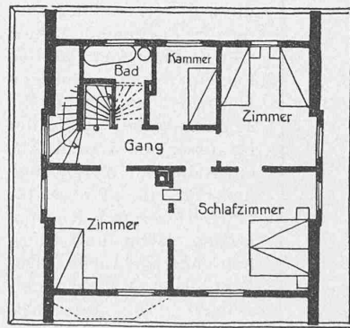
DACHGESCHOSS 2,80 m i. L.
