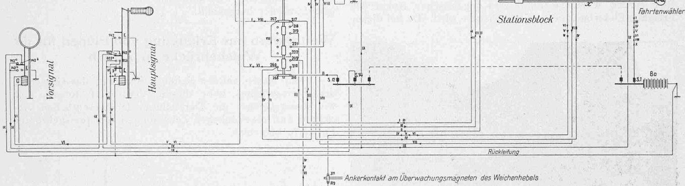
Abb. 15. Stromlaufanordnung der Fahrstrassen- und Signalschaltung.
