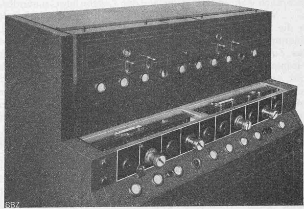
Abb. 13. Stationsblockwerk.
