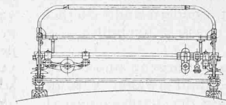
Abb. 27. Stromabnehmer. — 1:40.
